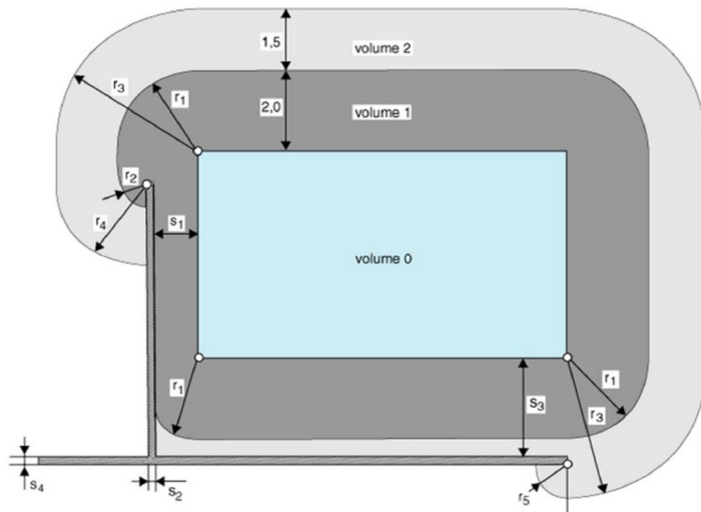
Figuur 23: bovenaanzicht zwembad met aanduiding volumes
