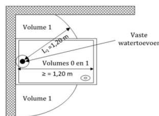
Figuur 18: Bovenaanzicht open douche met douchebak \geq 10 cm en breedte > 1,2 m
