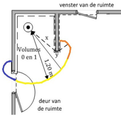
Figuur 14: Volumes bij douche zonder deur
