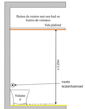
Figuur 13: dicht plafond
