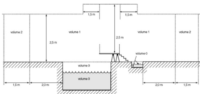
Figuur 25: doorsnede aanzicht verzonken zwembad / voetbad met verhoogd niveau en aanduiding volumes.
