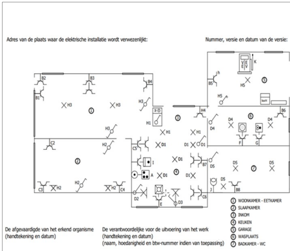
Figuur 37: Situatieplan van een huishoudelijke elektrische installatie
