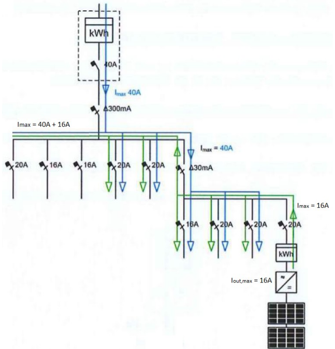
Figuur 29: Stroominjectie na bijkomende differentieel
