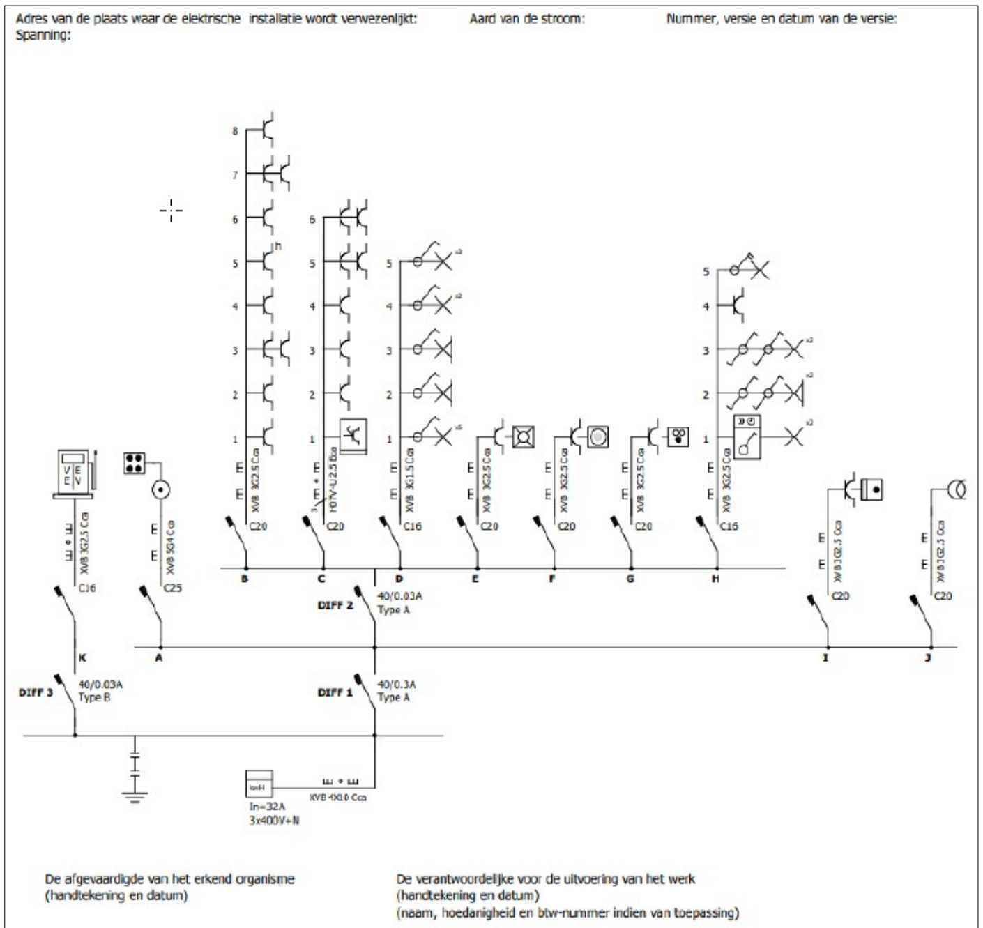
Figuur 36: Eéndraadschema van een huishoudelijke elektrische installatie
